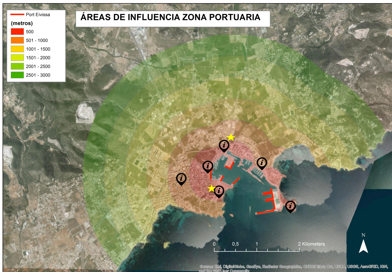
Figura 13. Localización aproximada de las estaciones de la red SmartSensPort-Eivissa
