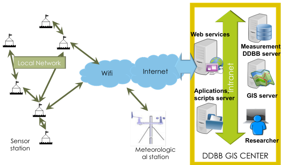
Figura 12. Arquitectura propuesta para la red SmartSensPort-Eivissa
