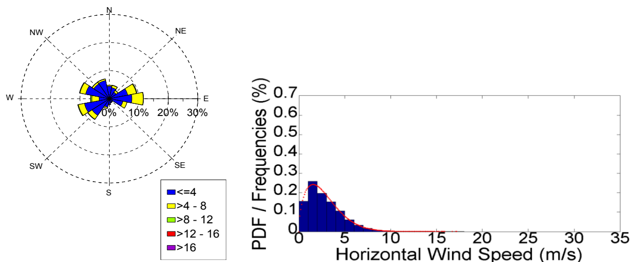
Figure 10. Rosa de vientos (Izda) y distribución de frecuencias de velocidad del viento (Dcha) para medidas 10 minutales tomadas en estación AEMET del Aeropuerto de Eivissa en el periodo 1989-2008.
