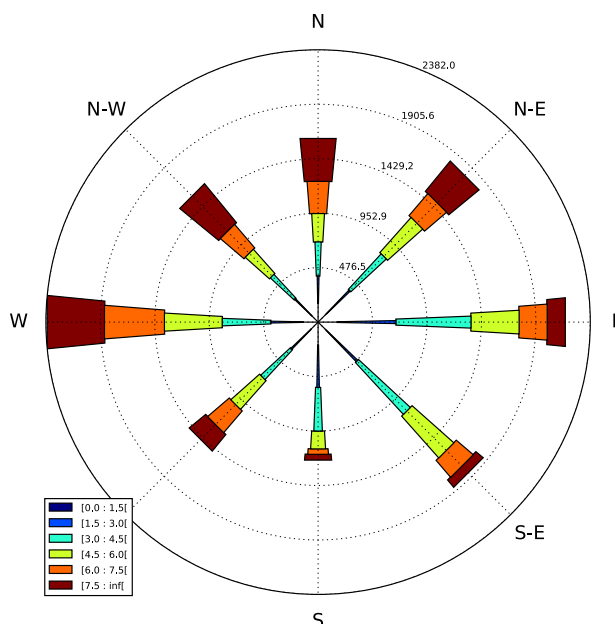
Figure 11. Rosa de los vientos extraída del modelo operacional de investigación MM5 sobre el punto de simulación del Port d'Eivissa. La escala de colores indica categorías de velocidad del viento (en m/s). La extensión radial de las aspas indica el número de registros en esa dirección y categoría de velocidad.
