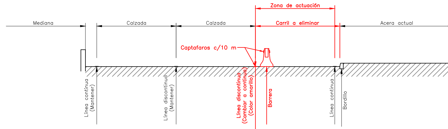
Sección tipo Tramo Monsenyor Palmer- S'Aigo Dolça
